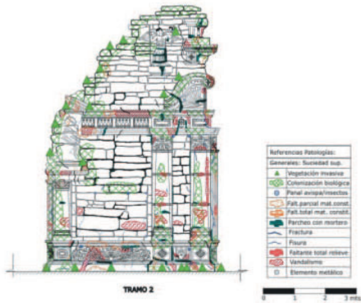
Figura 9. Relevamiento de deterioros de la Portada Principal de la Iglesia de San Ignacio Miní.
