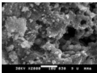
Fig. 4 (der). Detalle a mayor magnificación de la microestructura de la hematita (2000x).
