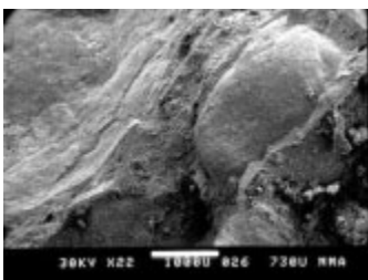
Fig. 4 (izq). Vista en MEB de una oolita de óxidos de hierro en el itacurú (22x).
