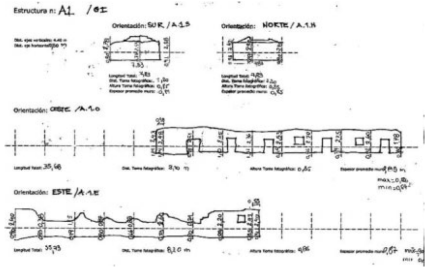
Figura 2. Ficha de apoio para o levantamento de dimensões e fotográfico da Estructura A.1.
