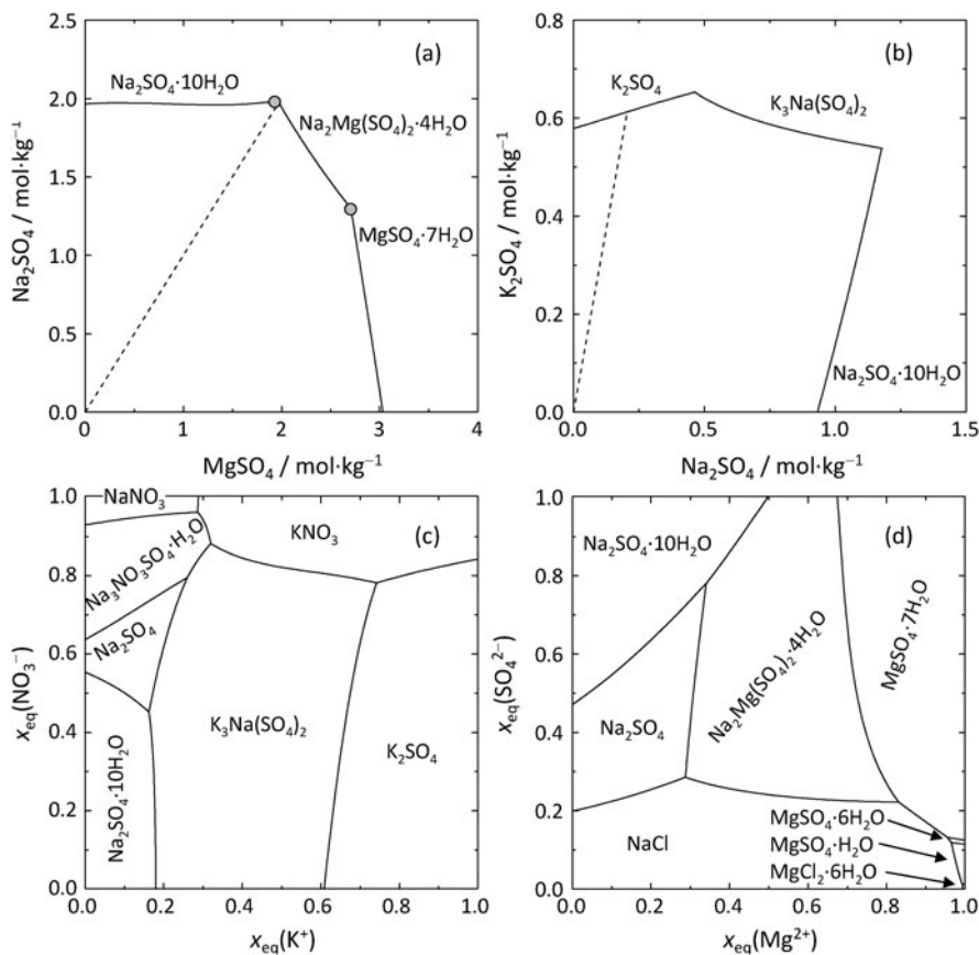
Fig. 4.28 Solubilities in (a) the \text{Na}_2\text{SO}_4\text{--MgSO}_4\text{--H}_2\text{O} system at 25^\circ\text{C} , (b) the \text{Na}_2\text{SO}_4\text{--K}_2\text{SO}_4\text{--H}_2\text{O} system at 15^\circ\text{C} , (c) the \text{Na}^+\text{--K}^+\text{--NO}_3^-\text{--SO}_4^{2-}\text{--H}_2\text{O} system at 25^\circ\text{C} , and, (d) \text{Na}^+\text{--Mg}^{2+}\text{--Cl}^-\text{--SO}_4^{2-}\text{--H}_2\text{O} system at 25^\circ\text{C}
