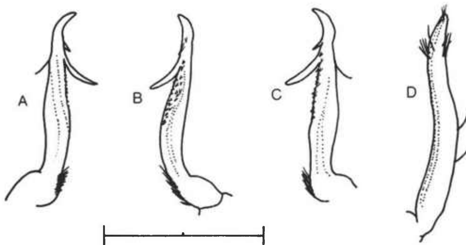
Fig. 8. Male right gonopod (first pleopod). A–C, Micropanope pusilla A. Milne Edwards: A, posterior view; B, mesiolateral view; C, anterior view; D, Dissodactylus juvenilis Bouvier, posterior view. Scale equals 1 mm.
