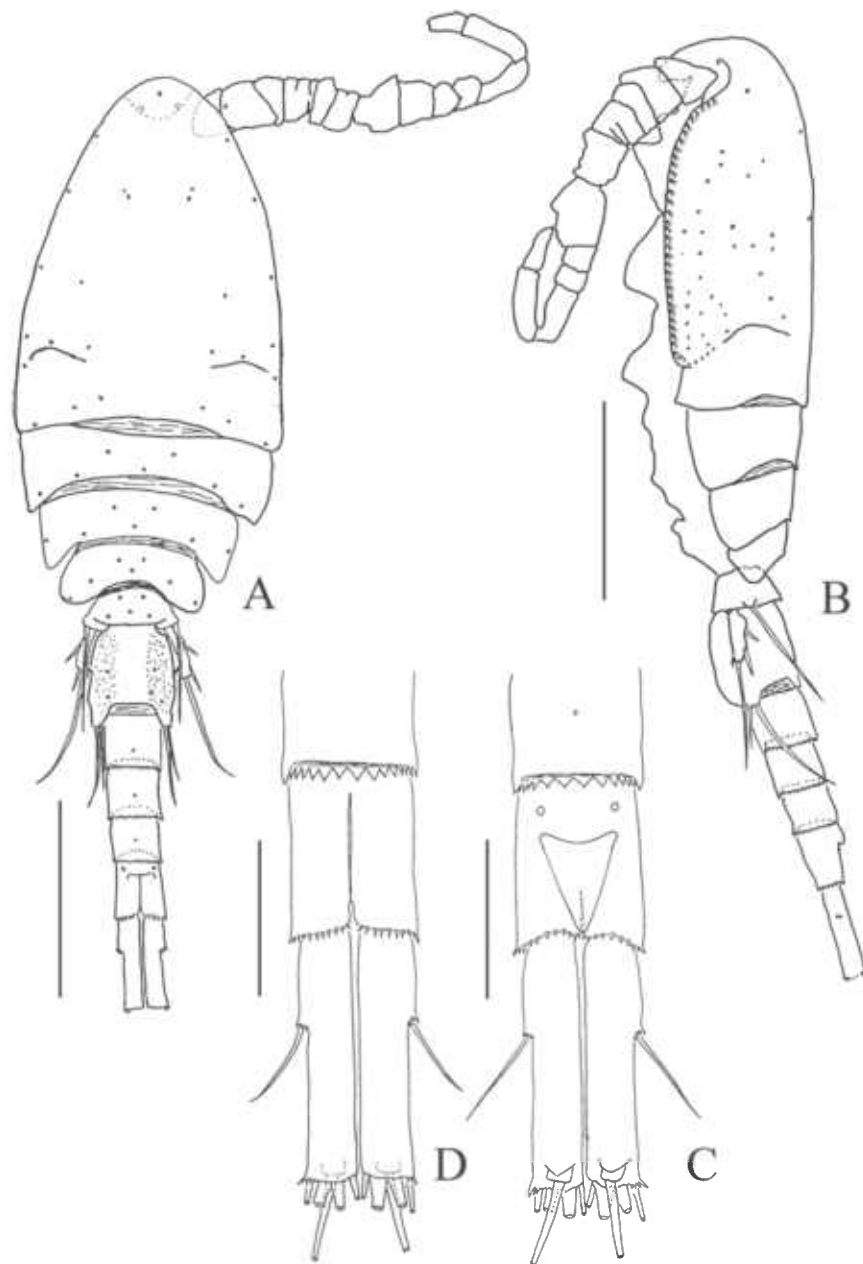
Fig. 6. Limnoithona tetraspina Zhang et Li, 1976. Male.
