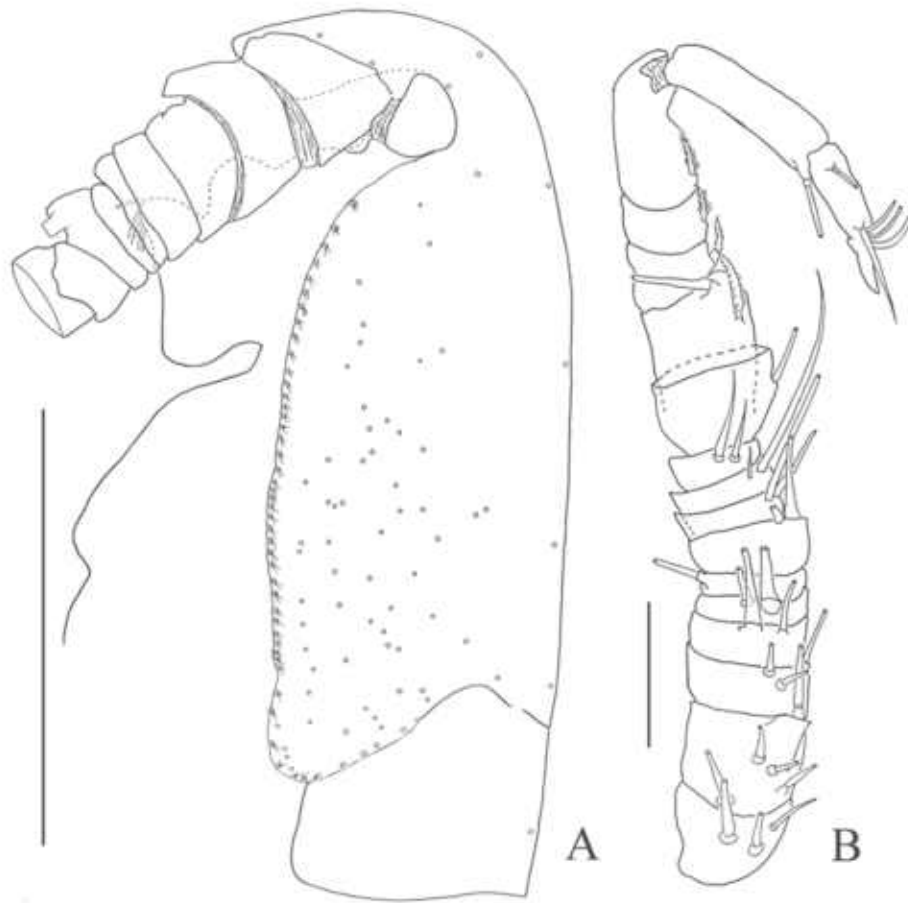
Fig. 7. Limnoithona tetraspina Zhang et Li, 1976. Male. A — cephalothorax, lateral; B — antennula. Scale bars: A — 0.10 mm; B — 0.025 mm. Fig. 7. Limnoithona tetraspina Zhang et Li, 1976. Самец: A — цефалоторакс, вид сбоку; B — антеннула. Масштаб: A — 0,10 мм; B — 0,025 мм.
