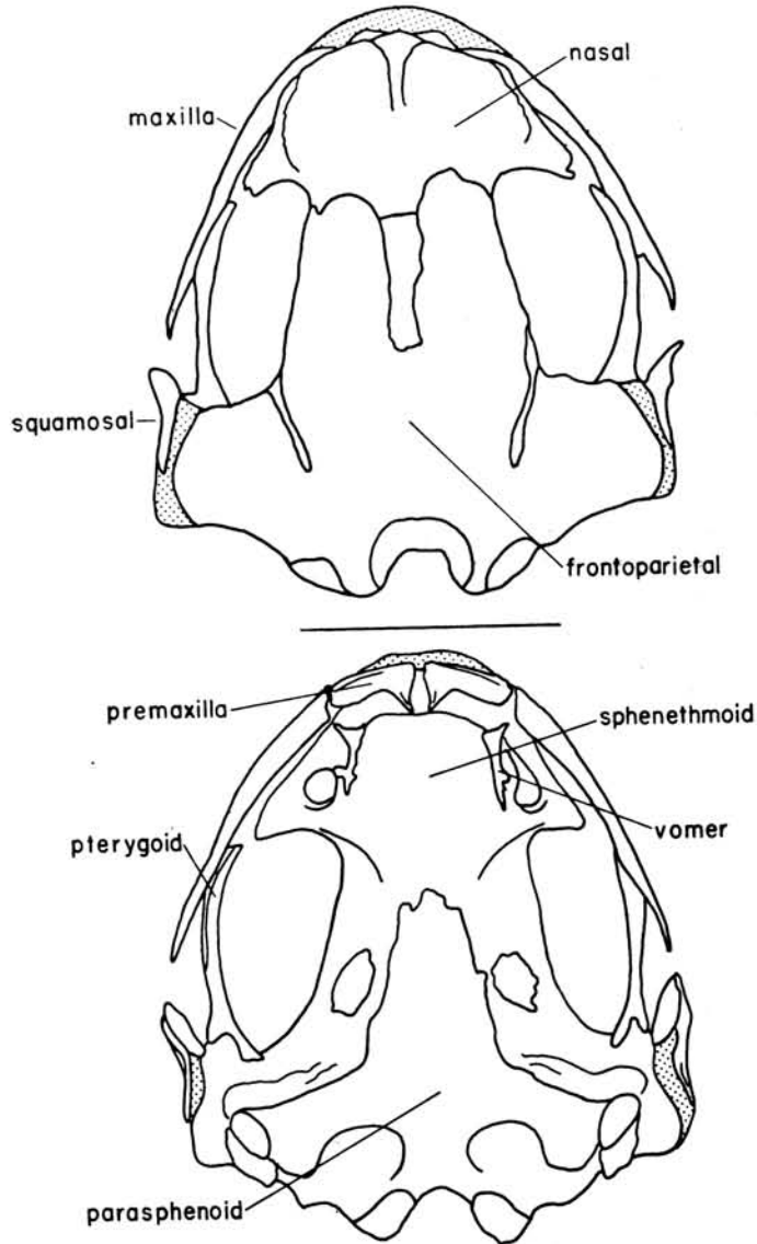
Fig. 1. — Vista dorsal y ventral del cráneo de Melanophryniscus rubriventris (Vellard), macho de 48 mm, de sierra de Calilegua, Jujuy, Argentina. Las áreas punteadas son cartilaginosas. Escala = 5 mm.
