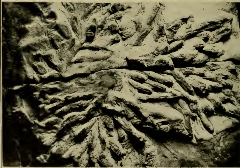
SSUYEN FORMATION
