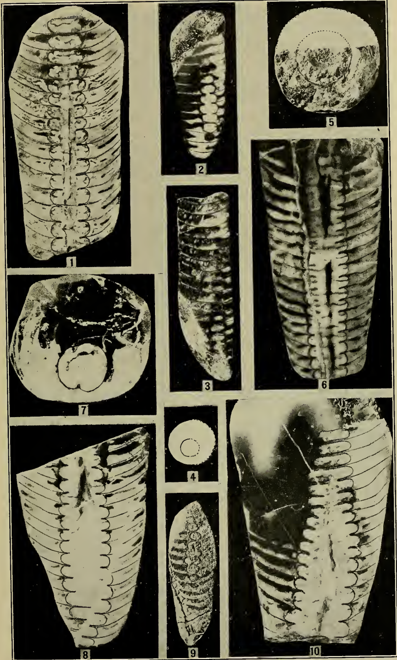
SSUYEN FORMATION
