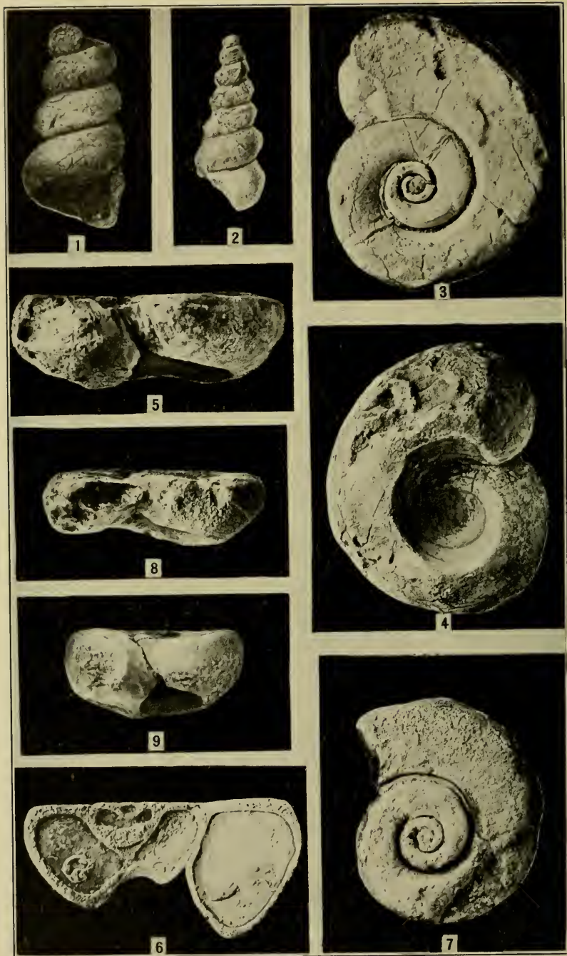
SSUYEN FORMATION
