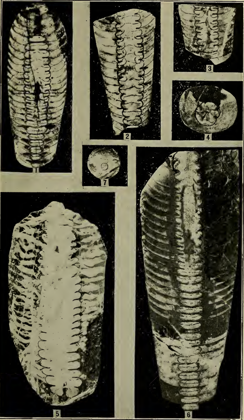
SSUYEN FORMATION
