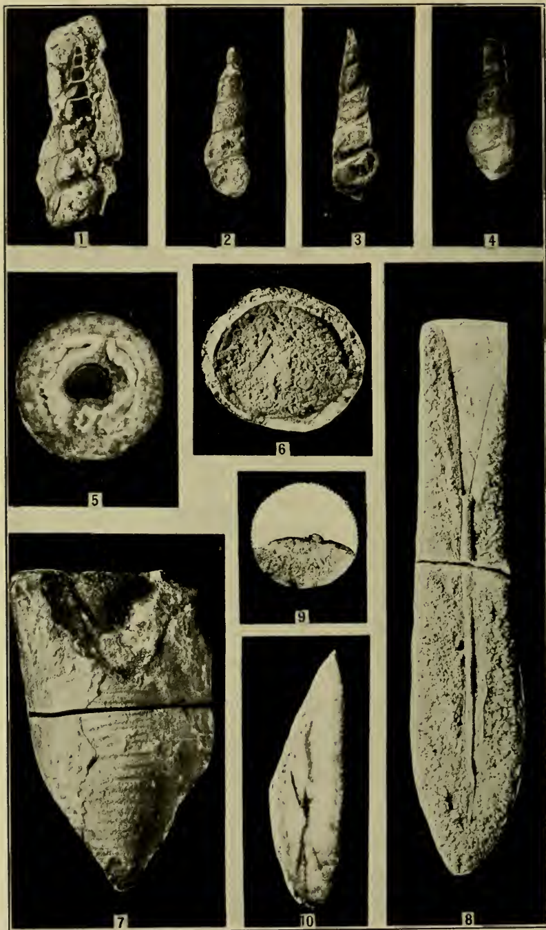
SANTAO FORMATION
