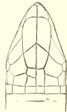
FIG. 133.—AMPHISBÆNA BAKERI, 2\frac{1}{2} \times natural size. Top of head. No. 25541, U. S. N. M.
