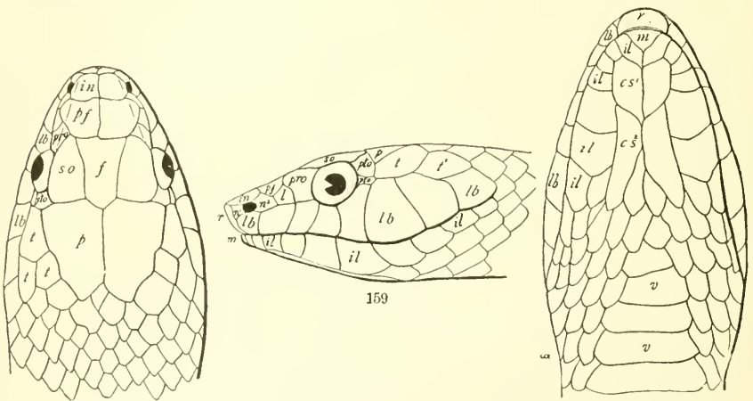
FIGS. 158-160.—HEAD-SHIELDS OF A CORONELLIDE SNAKE. cs 1 , anterior chin-shields; cs 2 , posterior chin-shields; f , frontal; il , lower labials; in , internasals; l , loreal; lb , supralabials; m , mental; n 1 , anterior nasal; n 2 , posterior nasal; p , parietal; pf , prefrontals; pro , preocular; pto , postocular; r , rostral; so , supraocular; t , temporals; v , ventrals.
