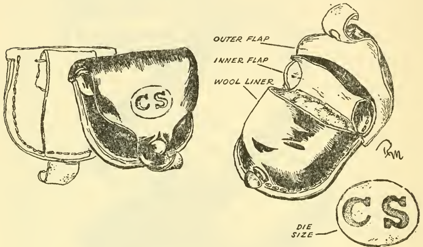
FIG. 15.—Confederate cap box. (R. L. Miller.)
