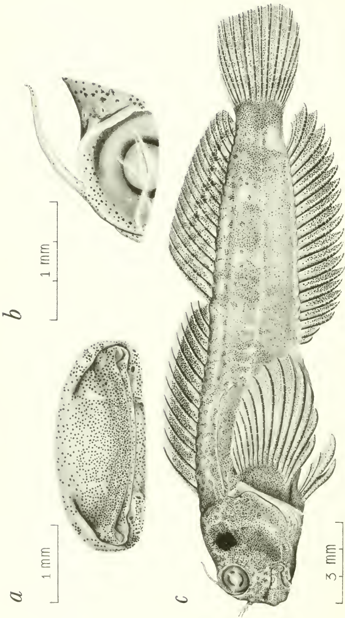
Entomacrodus macrospilus , USNM 200279, holotype, male, 18.7 mm SL, Marquesas Islands: a, upper lip; b, left supraorbital cirrus; c, lateral view.
