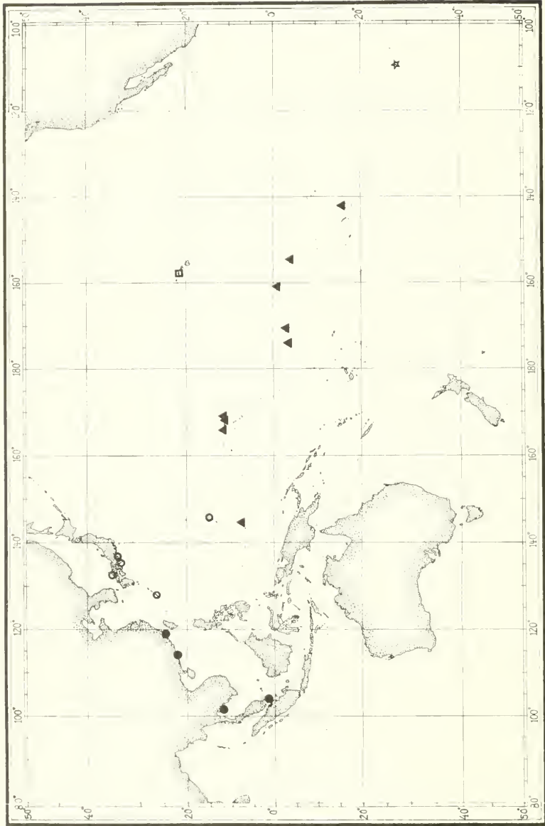
▲ E. cymatobiotus ◻ E. strasburgi ★ E. chapmani ● E. s. lightii ○ E. s. stelleri FIGURE 8.—Distribution of some species and subspecies of Entomacrodus .
