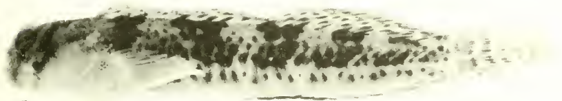
Entomacrodus marmoratus , USNM 197201, females, Oahu: a , 55.9 mm SL; b , 67.7 mm SL; Entomacrodus striatus , males: c , UH 03081, 54.7 mm SL, Tahiti; d , SU 62002, 54.0 mm SL. South China Sea.
