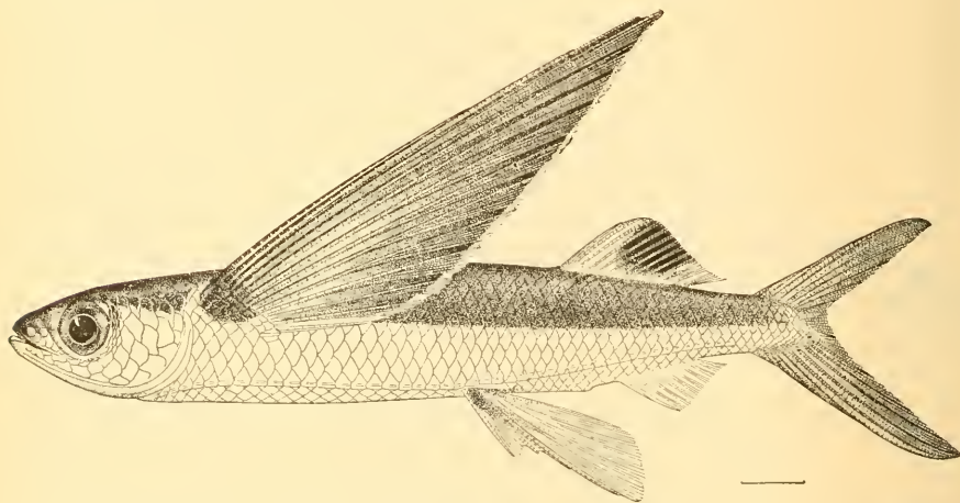
FIG. 2.—CYPSILURUS SPILONOPTERUS.
