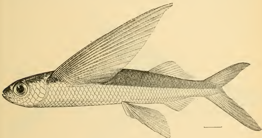
FIG. 1.— CYPSILURUS OGILBYI .
