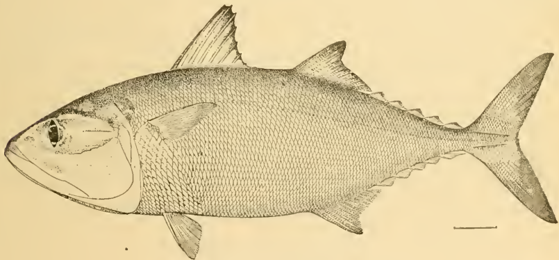
FIG. 3.—RASTRELLIGER BRACHYSOMUS.
