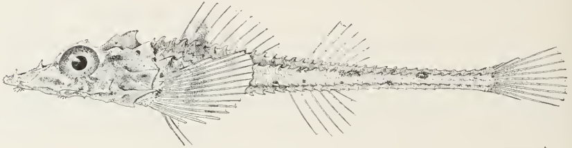
FIG. 11.— PODOTHECUS THOMPSONI .
