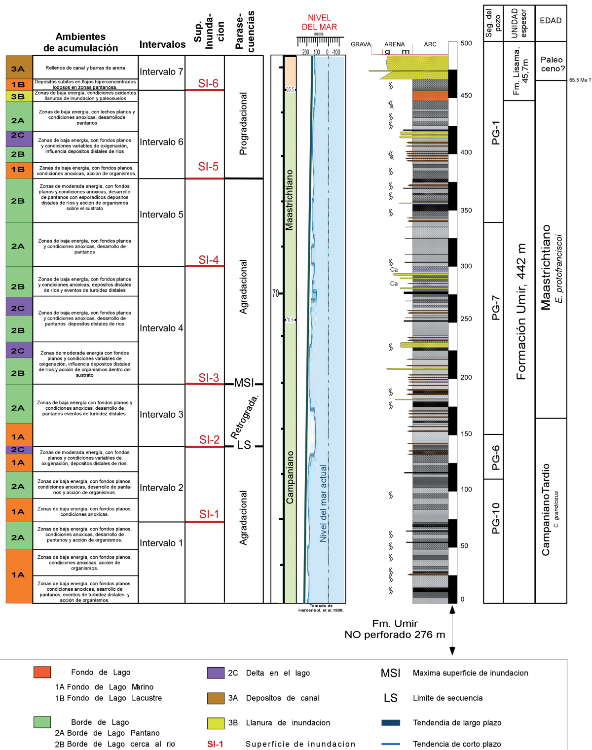
FIGURA 5. (páginas izquierda y derecha). Columna estratigráfica generalizada del segmento superior de la Formación Umir y base de la Formación Lisama, indicando las superficies de inundación (SI) identificadas, la ocurrencia de la materia orgánica amorfa y de Pediastrum sp., y el análisis de ambientes de acumulación y de secuencias estratigráficas.
