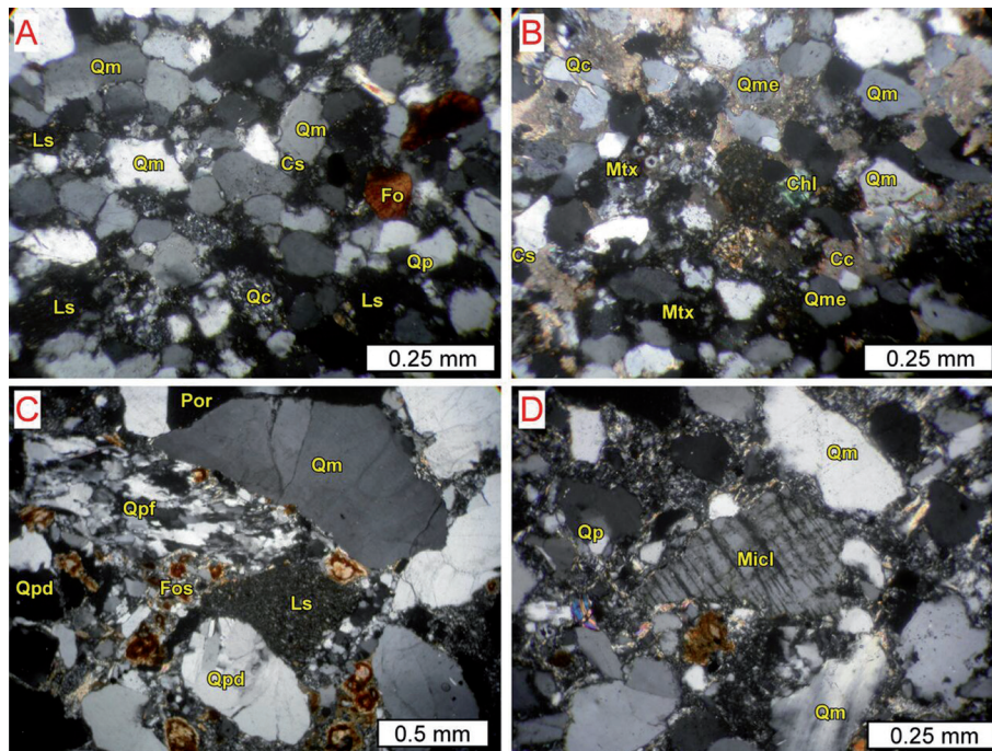
FIGURA 8. Fotomicrografías de sección delgada a 10X con nicóles cruzados. A. Sección PG7-60 (Formación Umir), con granos de cuarzo monocristalino (Qm), algunos con sobrecrecimiento de sílice (Cs), cuarzo policristalino (Qp), chert (Qc), líticos sedimentarios (Ls) y fragmentos de fósiles (Fo). B. Sección PG7-184.5 (Formación Umir) ilustrando el predominio de cuarzo monocristalino (Qm) con sobrecrecimiento de sílice, cuarzoesudrales (Qme), cloritas (Chl), y formas de oolitos síliceos en la matriz (Mtx). C. Sección PG1-19.3 (Formación Lisama), fotos tomadas a 4X, con abundante contenido de cuarzo policristalino, difuso y foliado (Qpd, Qpf), y líticos sedimentarios (Ls). También se encuentran algunos fósiles (Fos, ostrácodos?) en la matriz. D. Sección PG1-12.0 (Formación Lisama), fragmento de microclina (Micl).
