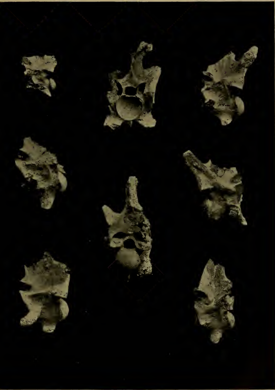
VERTEBRÆ OF PTEROSPHEMUS SCHUCHERTI.
